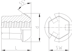
tuerca asiento esférico 55° con ranuras de inyección domed nut 55° with grout slots
