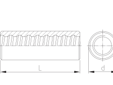
manguito estándar coupler standard
