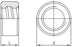
SAS SYSTEMS tuerca de fijación fix ring
