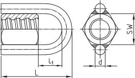
tuerca hexagonal con argolla ring nut
